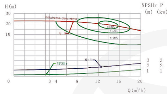
SCP-10 (Q-H曲線圖/Graph)
