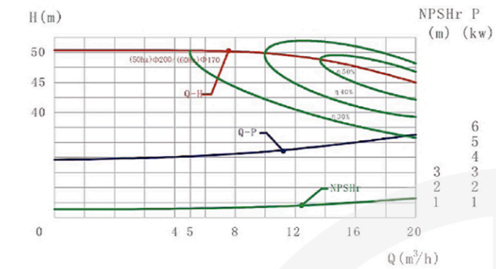
SCP-25 (Q-H曲線圖/Graph)
