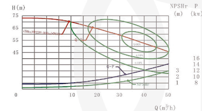
SCP-35-1 (Q-H曲線圖/Graph)
