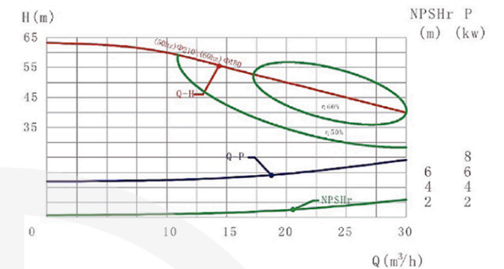
SCP-30 (Q-H曲線圖/Graph)
