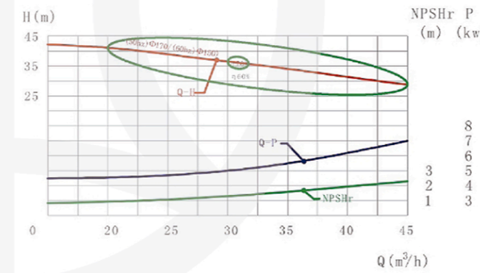
SCP-20-2 (Q-H曲線圖/Graph)
